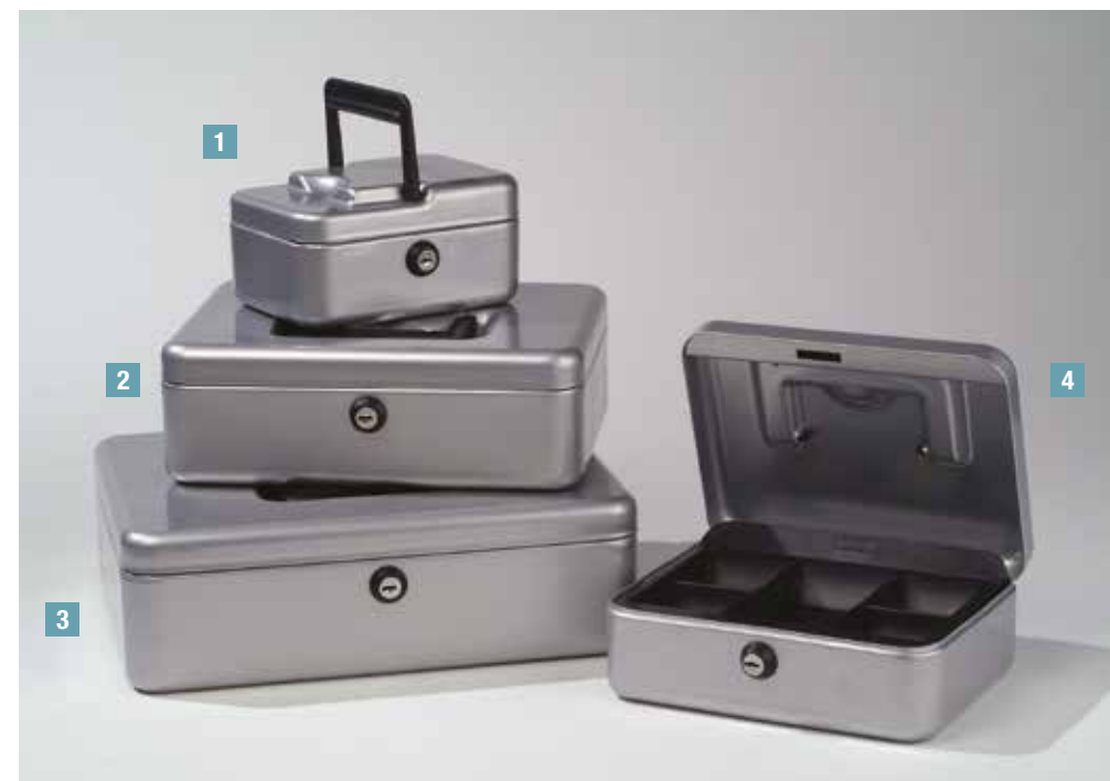
1 Boîte à monnaie - 15 cm : Épaisseur de tôle : 10/10 ème Dim. : L.15,5 x H.8 x P.11 cm
